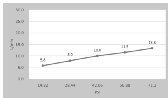
Curva de caudal.
