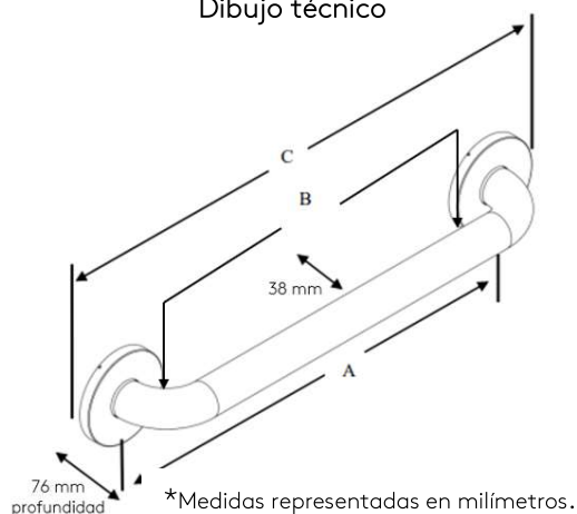
Dibujo técnico
